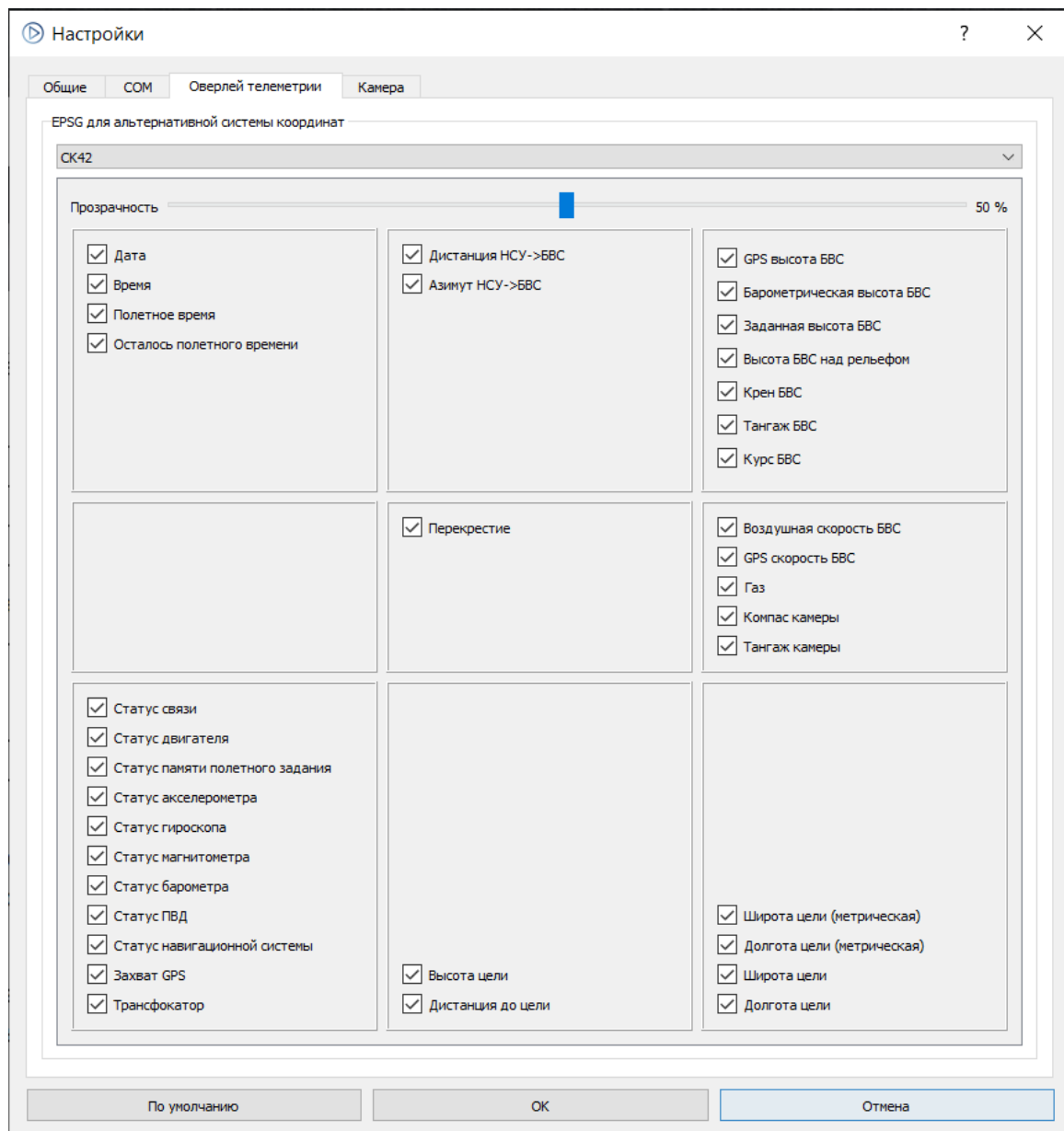
Рисунок 20 – Вкладка «Оверлей телеметрии» окна «Настройки»
