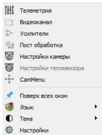
Рисунок 9 – Подменю «Окно»
