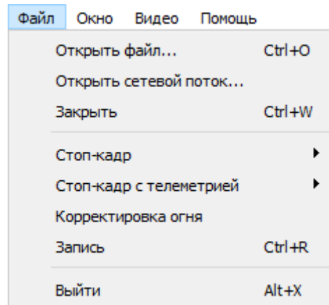
Рисунок 3 – Подменю «Файл»
