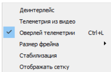
Рисунок 22 – Подменю «Видео»
