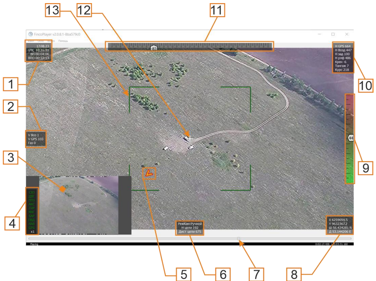
Рисунок 23 – Окно видеоинформации
