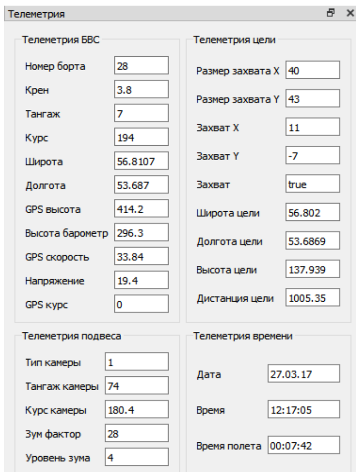
Рисунок 10 – Окно «Телеметрия»
